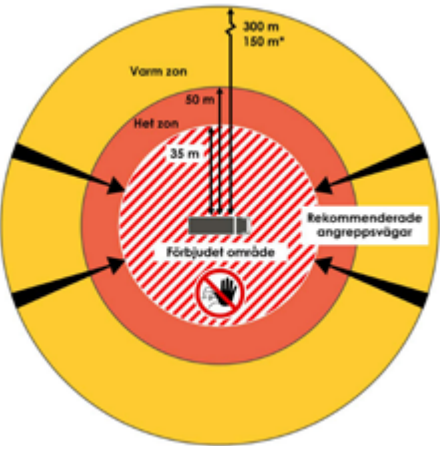
LNG, tung lastbil, tryckkärlexplosion (ovanifrån)
