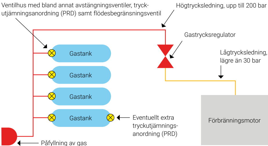
Principskiss över gassystemet i ett fordon som drivs med CNG (tryckkomprimerad metan).
